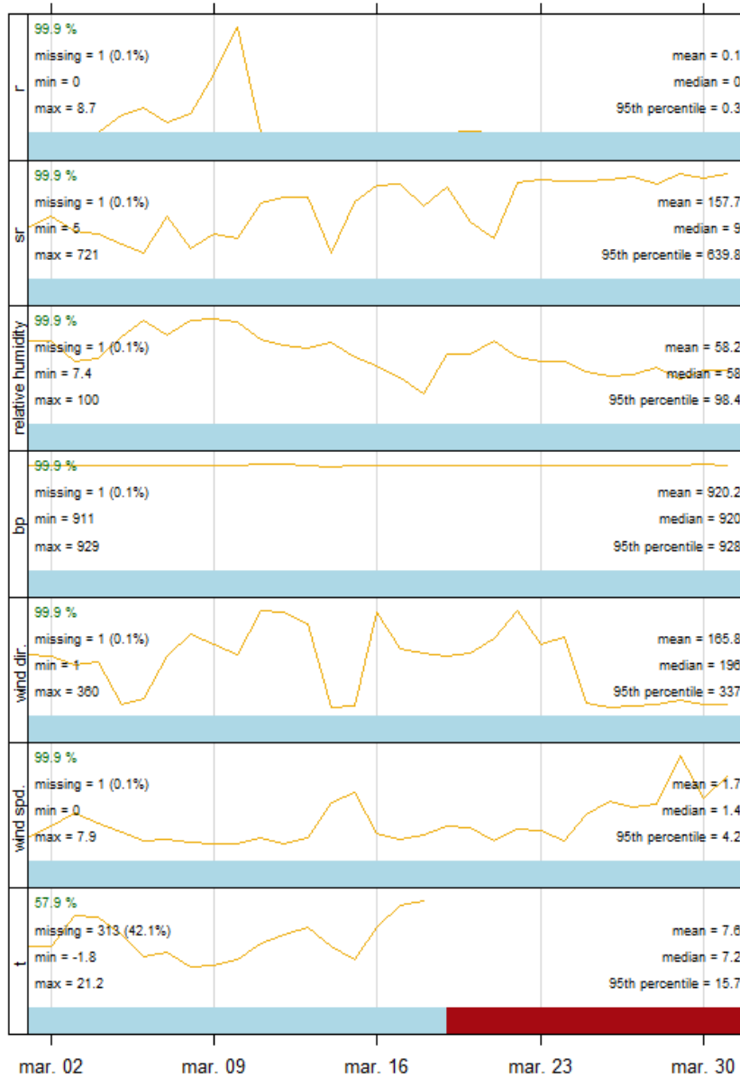
Estación de cuenca - Evolución mensual, Marzo de 2026
