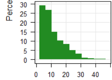
Histogramas
