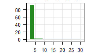
Histogramas
