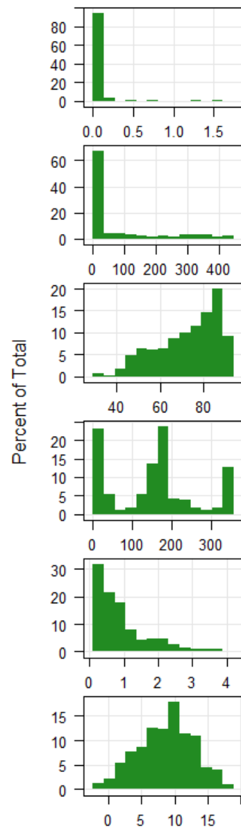
Histogramas
