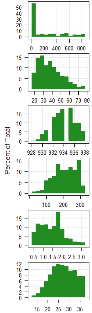
Histogramas
