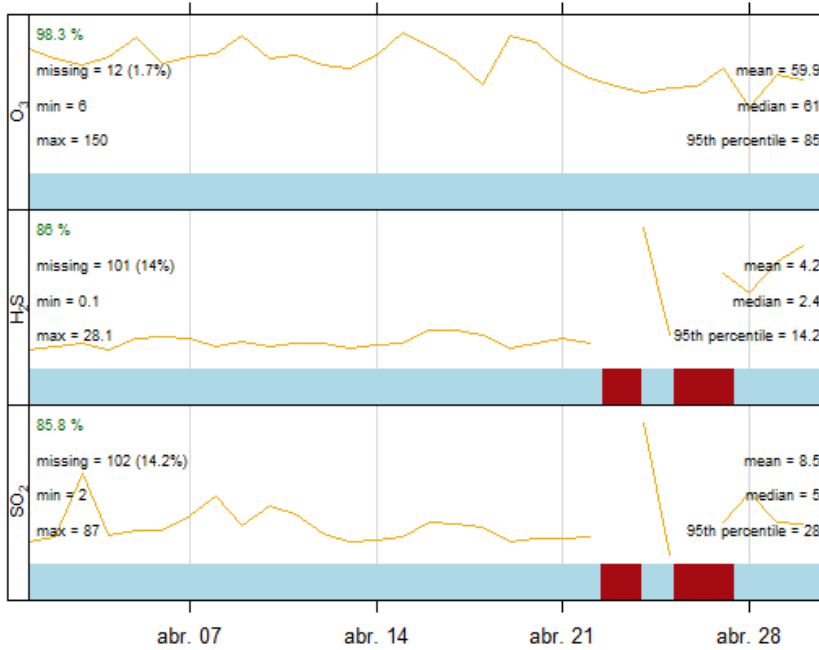
Estación de Rampas mecánicas - Evolución mensual, Abril de 2025
