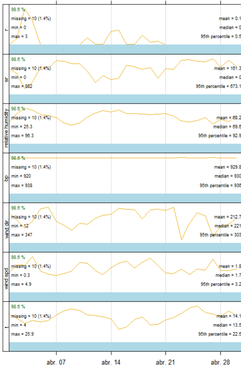
Estación de Rampas mecánicas - Evolución mensual, Abril de 2025
