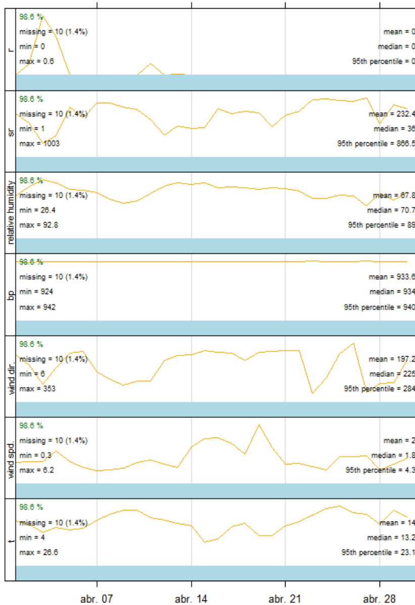
Estación de Almacén municipal- Evolución mensual, Abril de 2025
