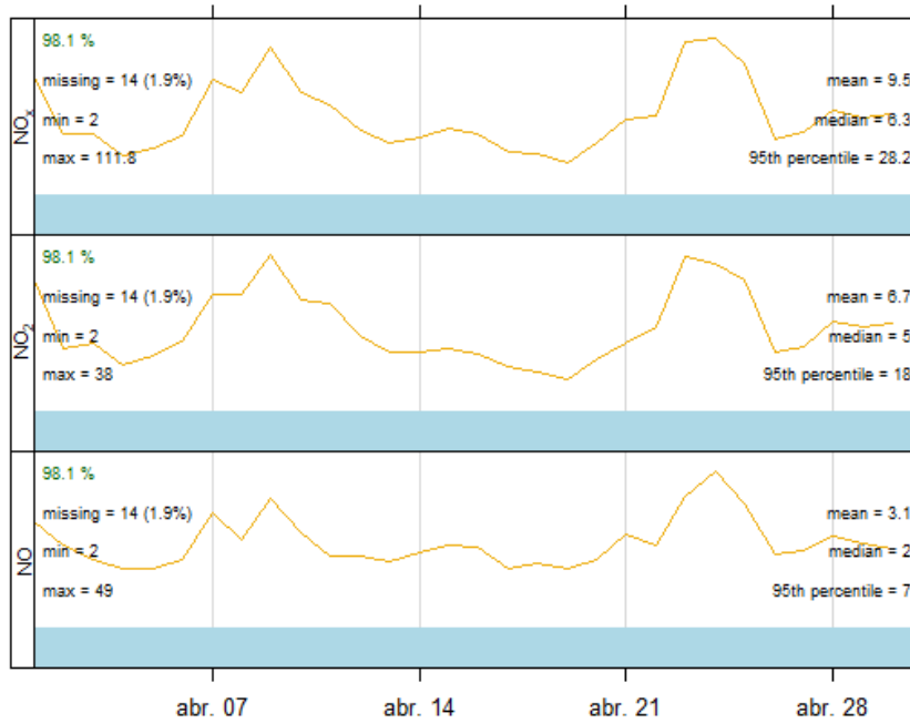
Estación de Almacén municipal- Evolución mensual, Abril de 2025
