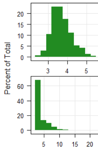
Histogramas
